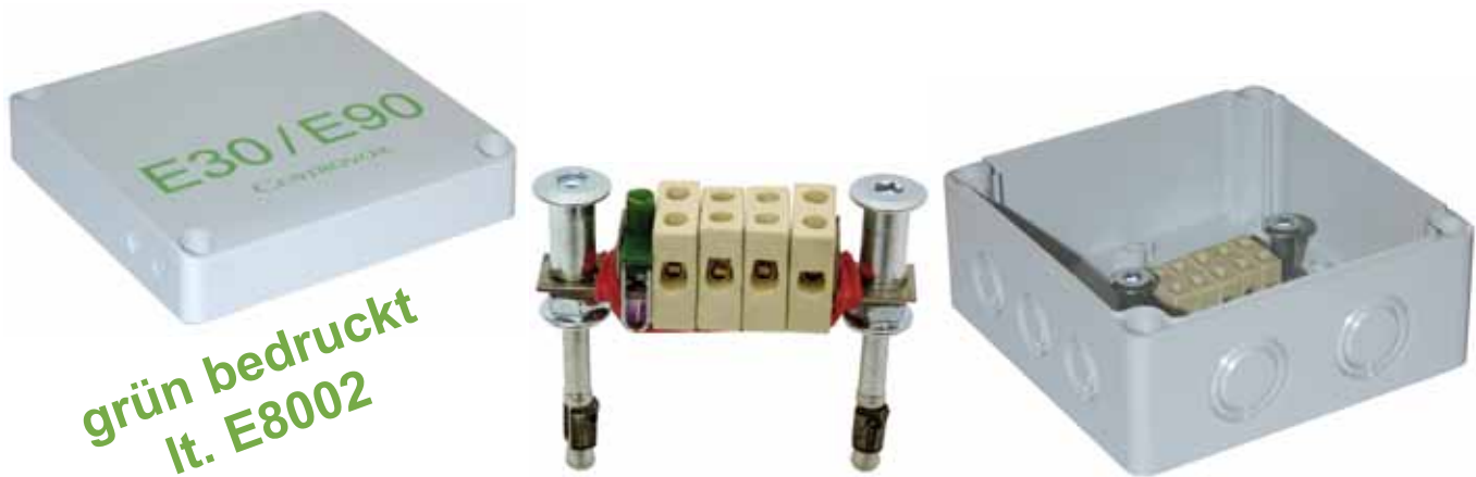
5 Klemmen 4mm 2
