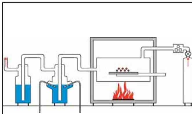
Korrosivität der Brandgase IEC 60754-2, ÖVE/ÖNORM EN 50267-2-2
