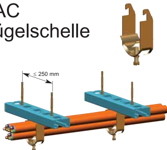
Verlegeabstand: ≤ 1.200 mm
