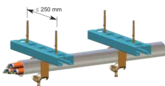
Verlegeabstand: \leq 1.200\text{ mm}
