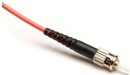
ST-Stecker straight tip (= Bajonett) (auch BFOC-Stecker genannt)
