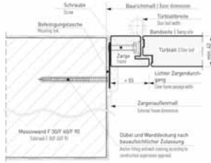
Detail flächenbündiger Einbau
