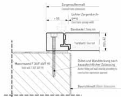
Detail „Auf Wand Montage“
