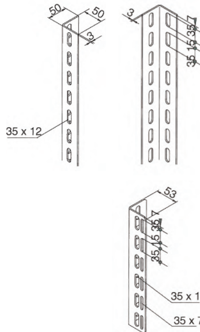
L-Profilschiene A4 50x50x3000
