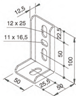
Winkel universal A4
