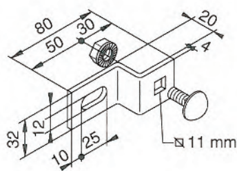
Steigleitungswandbügel A4 inkl. Schraubgarnitur M10x25
