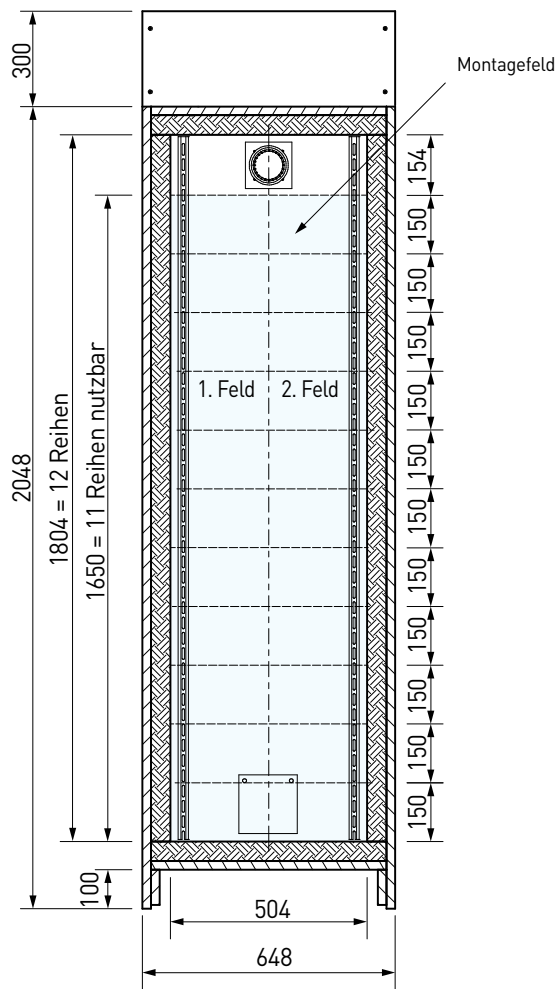
Nutzbare Innenraum am Beispiel eines PRIOELEC ESL91.12224
