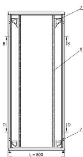
Vorderansicht Schranksiefe 800 mm
