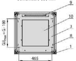
Schnitt C-C Schranksiefe 600 mm
