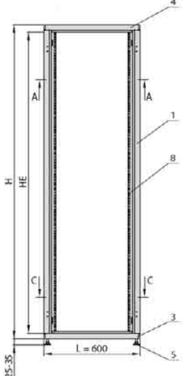
Vorderansicht Schranksiefe 600 mm
