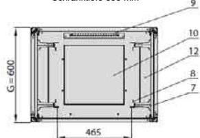
Schnitt D-D Schranksiefe 600 mm
