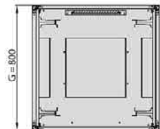
Schnitt D-D Schranksiefe 800 mm
