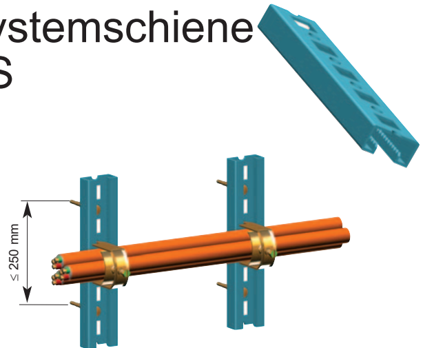
Verlegeabstand: ≤ 1.200 mm
