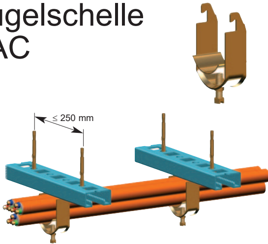
Verlegeabstand: ≤ 1.200 mm
